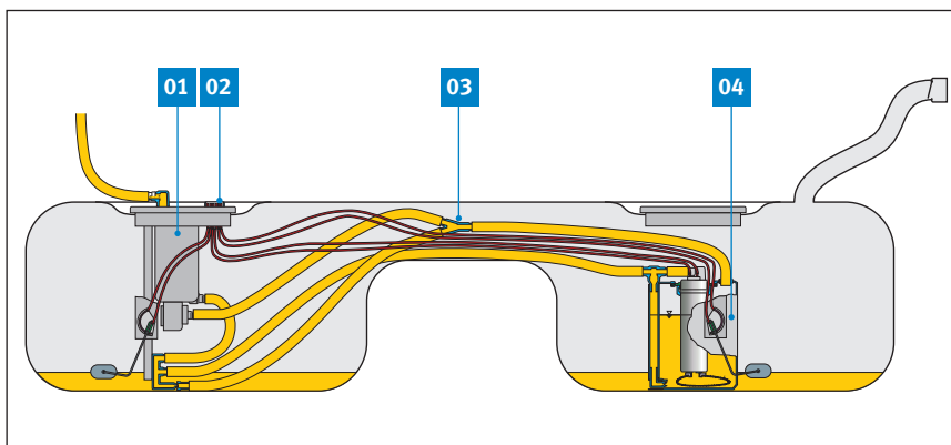
Рис. 3. Топливный бак в разрезе (схематическое изображение)
